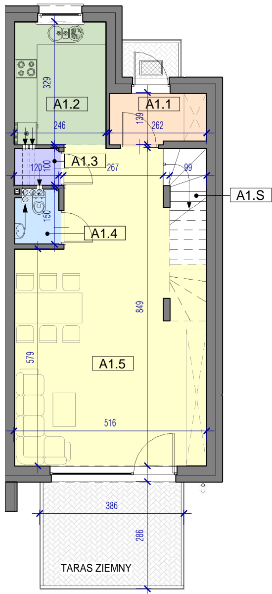
BUDYNEK NR 1 - RZUT PRZYZIEMIA
