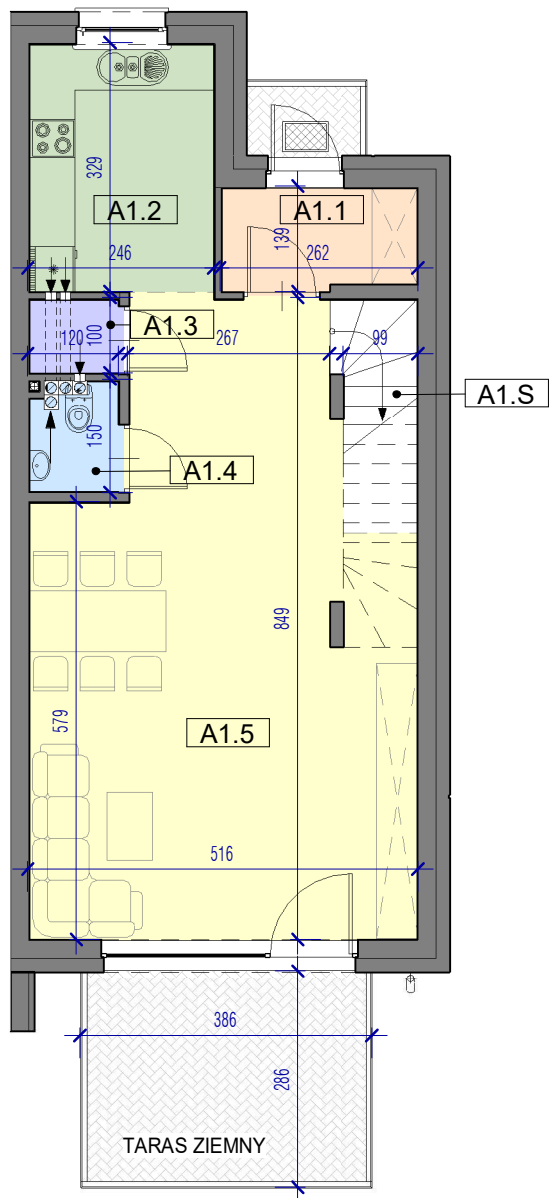
BUDYNEK NR 3 - RZUT PRZYZIEMIA
