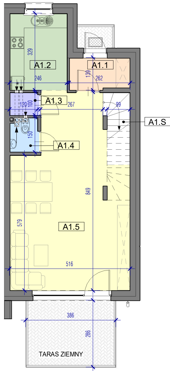
BUDYNEK NR 7 - RZUT PRZYZIEMIA
