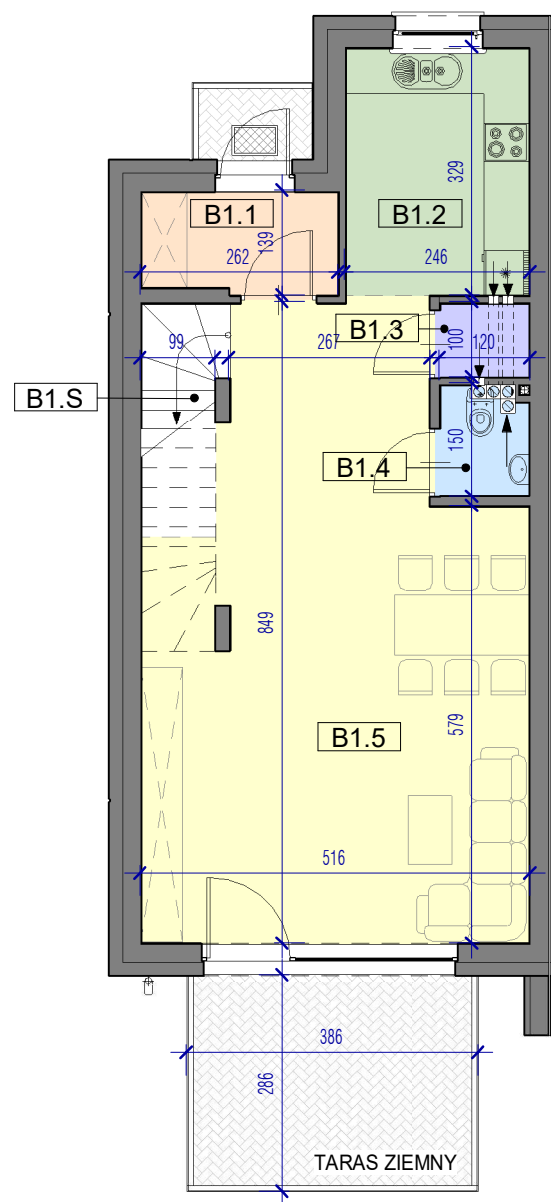
BUDYNEK NR 8 - RZUT PRZYZIEMIA 1 : 100
